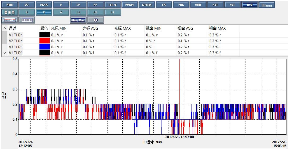
V1 THDr、V2 THDr、V3 THDr 分别为 A、B、C 相电压总畸变率
