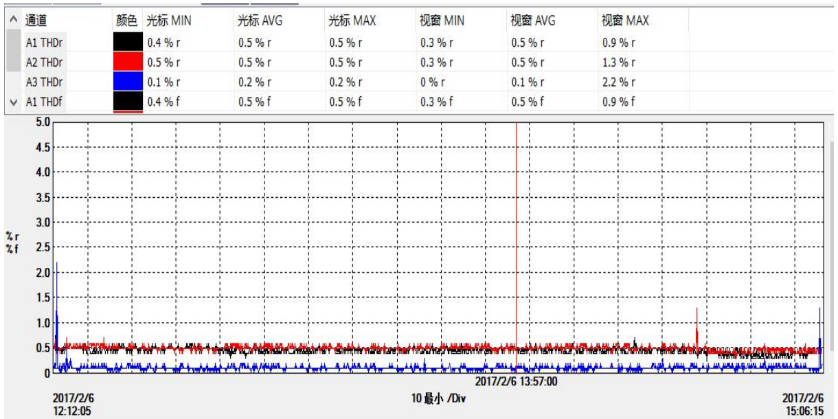
A1 THDr、A2 THDr、A3 THDr 分别为 A、B、C 相电流总畸变率
